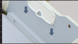
ランチングホイール 取り付け穴
