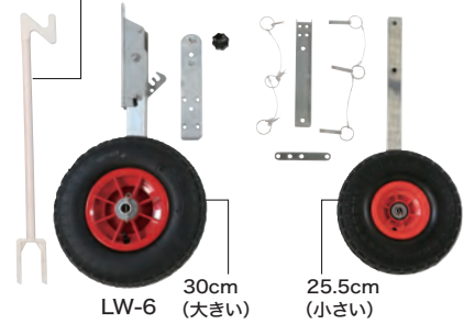
左がジョイクラフトの商品構成。右の他社製に比べ、シンプル構造なので作動は圧倒的に簡単、パーツ類も紛失しにくい仕様です。
